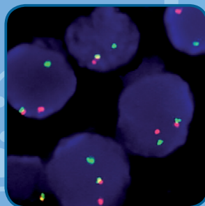
MYC
