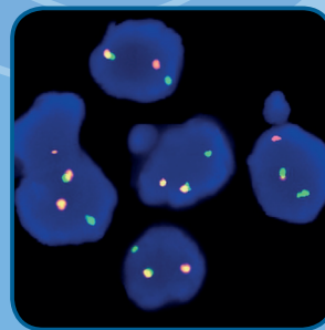
IGH
