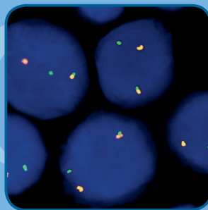
ALK
