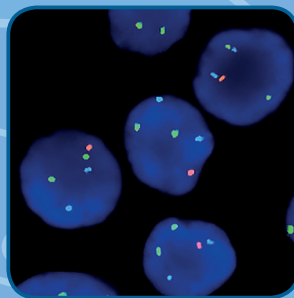
D13S319/13q34/CEN 12
