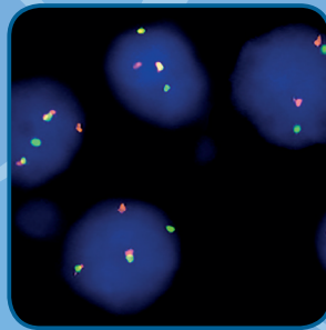
BCL2
